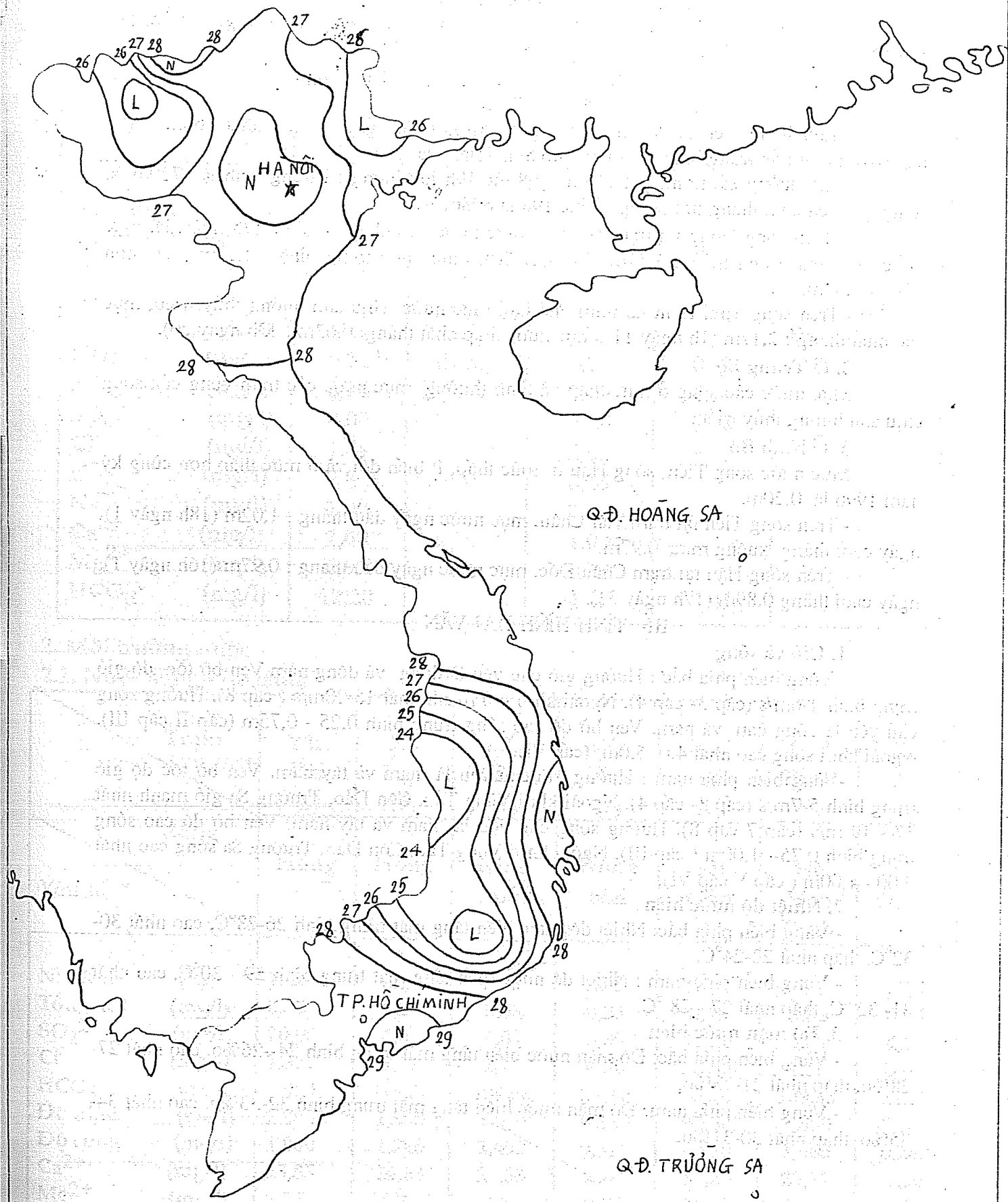
Hình 2. Bản đồ nhiệt độ trung bình tháng V năm 1997
