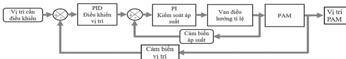
Hình 2. Cấu trúc Bộ điều khiển PID-PI
